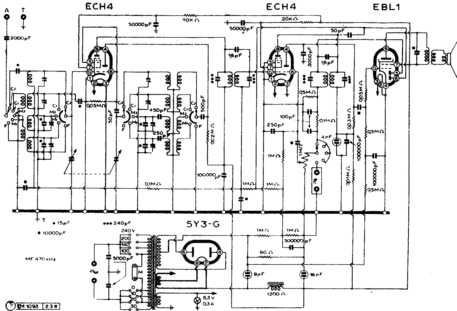
F.I.M.I. - MOD. PHONOLA « 417 »
